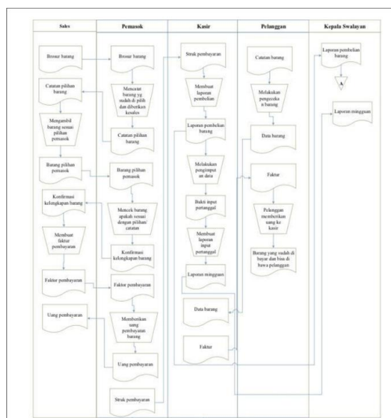
Gambar 1. Arsitektur Flowchart Sistem Informasi Terintegrasi Swalayan Aman
